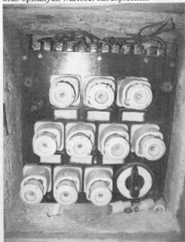
Foto nr 4 – widok rozdzielnic na I piętrze biblioteki – brak schematu elektrycznych połączeń oraz opisanych wartości zabezpieczeń.
